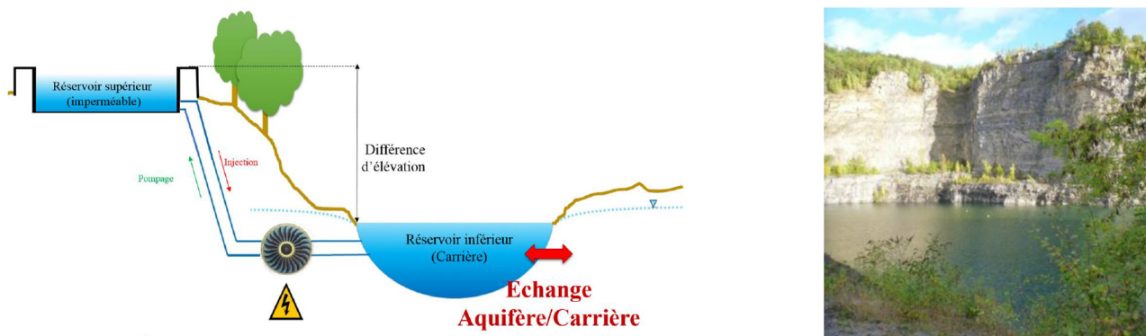
Fig. 2. Représentation simplifiée du concept de STEP en carrière (à g.) et exemple de la carrière de Maizeret en Belgique (à d.) (Poulain, 2018).
