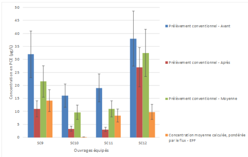
Figure 1 : Comparaison des concentrations en PCE dans les eaux souterraines (prélèvement conventionnel et concentration moyenne calculée, pondérée par le flux, pour les EPF)
