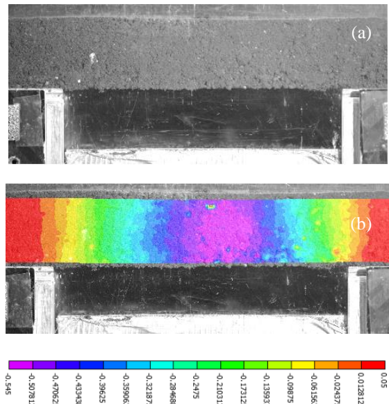
Figure 5. (a) Couche de sol naturel de hauteur H=5 cm non renforcée (b) Déplacement vertical (en mm) de la couche de sol avant le chargement
