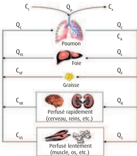
FIGURE 1 EXEMPLE DE DESCRIPTION SCHÉMATIQUE D'UN MODÈLE PBPK L'organisme est représenté par une série de compartiments, interconnectés par les flux sanguins et aériens, dont l'intensité est représentée par le paramètre Q, et la concentration en substance par le paramètre C.
