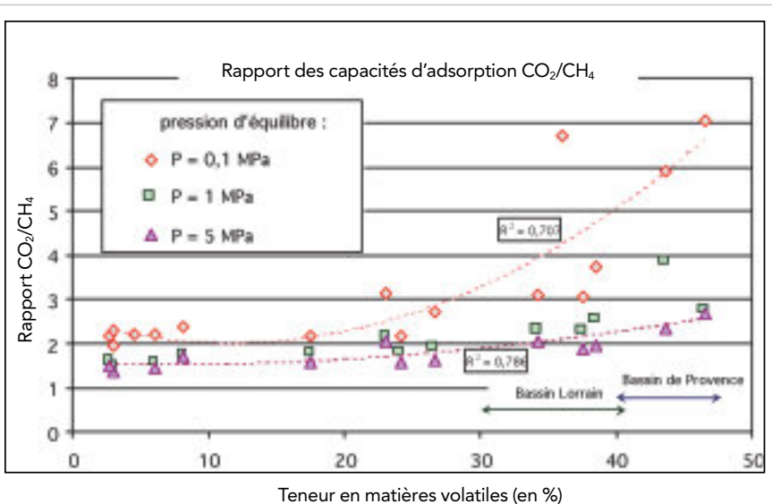
Relation entre la capacité d'adsorption du CO 2 et du méthane pour certains charbons français en fonction de leur teneur en matières volatiles.
