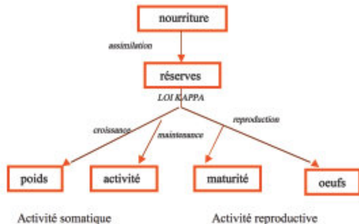
Représentation schématique de la répartition de l'énergie dans la théorie DEB.
