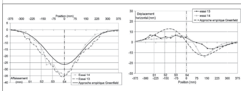
Déplacements en surface pour les essais en présence de la maquette de structure.
