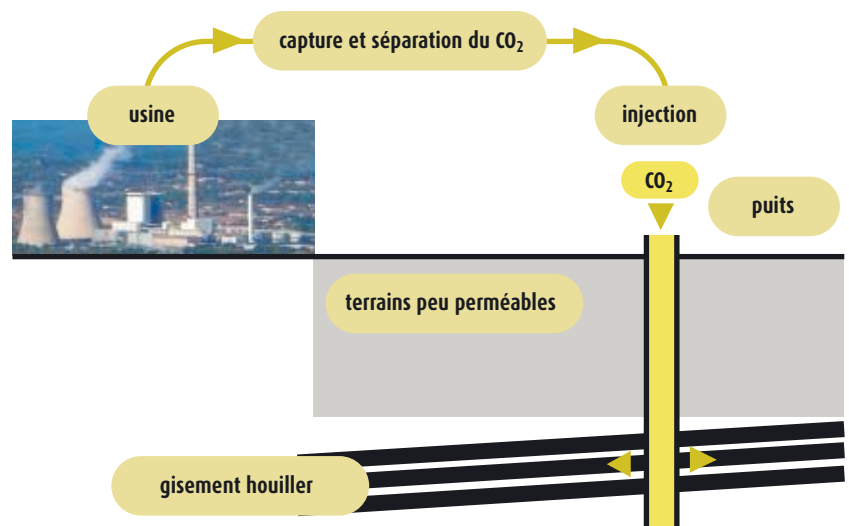
FIGURE 1. Schéma de principe de la récupération et du stockage du CO 2 dans les terrains houillers à l'échelle locale.
