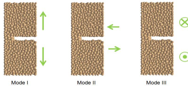
Figure 2. Modes de sollicitation et types de rupture associés
