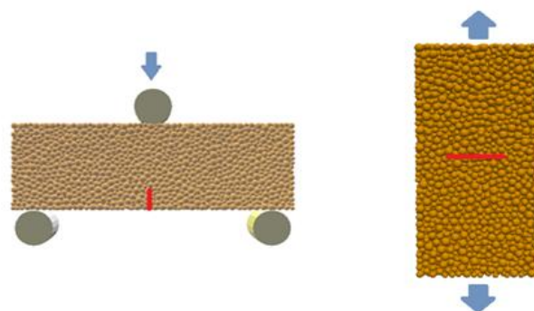
(b) Essai de traction directe sur un échantillon pré-fissuré de dimensions 20x40x20 cm 3
