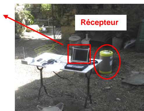
Figure 9 : Dispositif UGPS en surface
