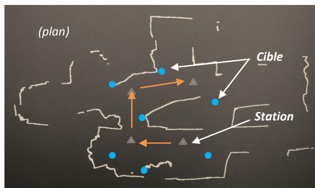
Figure 13 : Installation du scanner laser 3D en souterrain (cheminement vu en plan)
