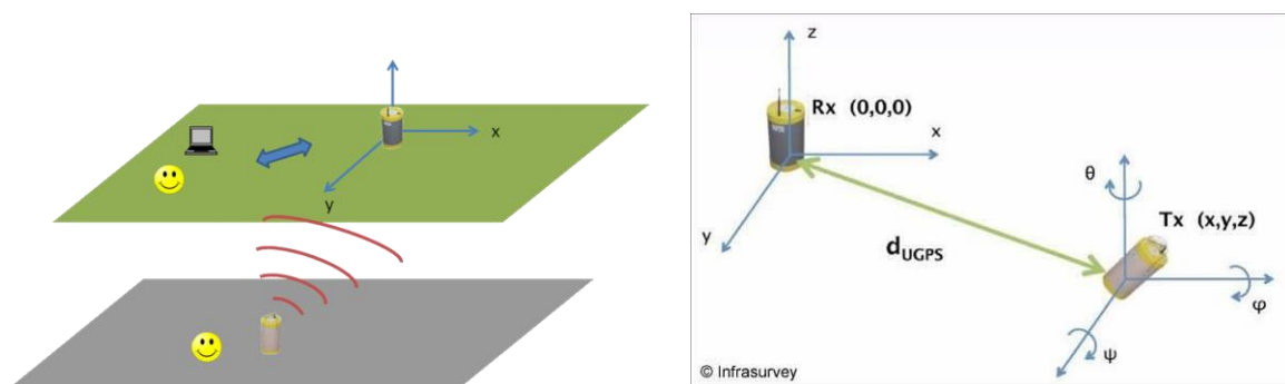
Figure 1 : Illustrations du principe de fonctionnement du système UGPS
