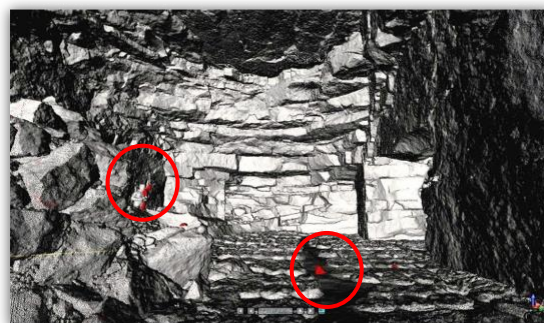
Figure 16 : Détection d'une chute de blocs
