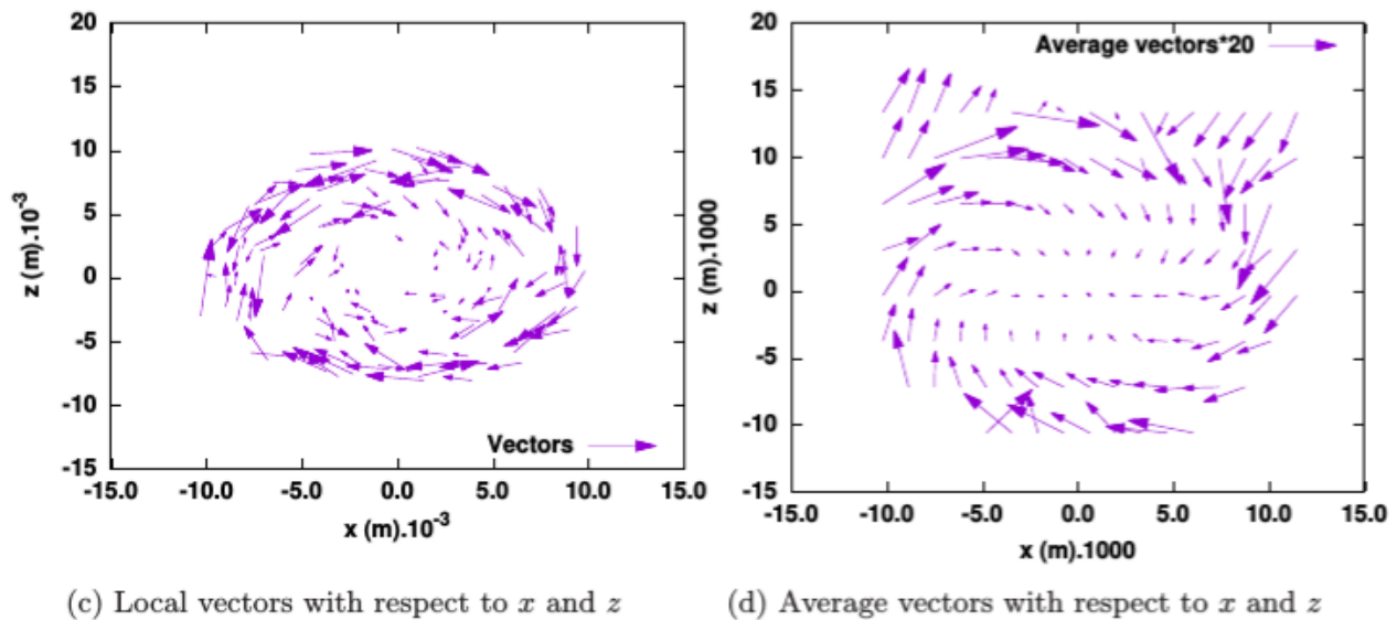
Figure 4: Mouvements instantanés et mouvements moyens de la particule dans le plan horizontal. Moyennes produites par rapport au temps t et à la hauteur y .
