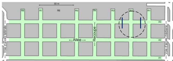
Figure 3: Zoomed-in image of pillars, aisles and intersections and location of cracks (blue) (MDPA, 2015). Key: Voie d'accès latérale - Side access route; Voie d'accès médiane - Middle access route; allées - aisles; recoupe - intersection; R1, R2... - I1, I2...
