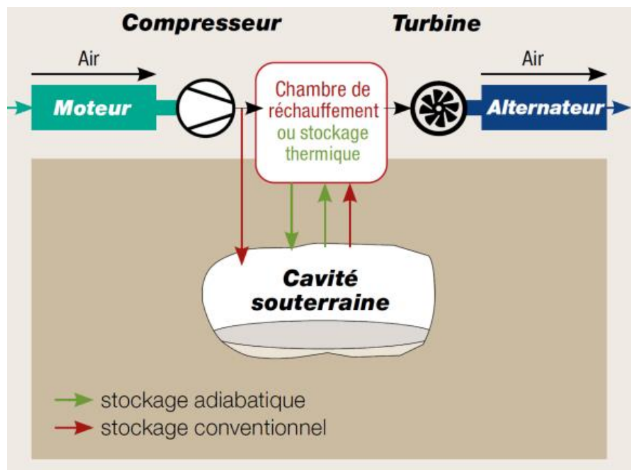
Figure 6. Schéma simplifié des installations d'un stockage souterrain d'air comprimé
