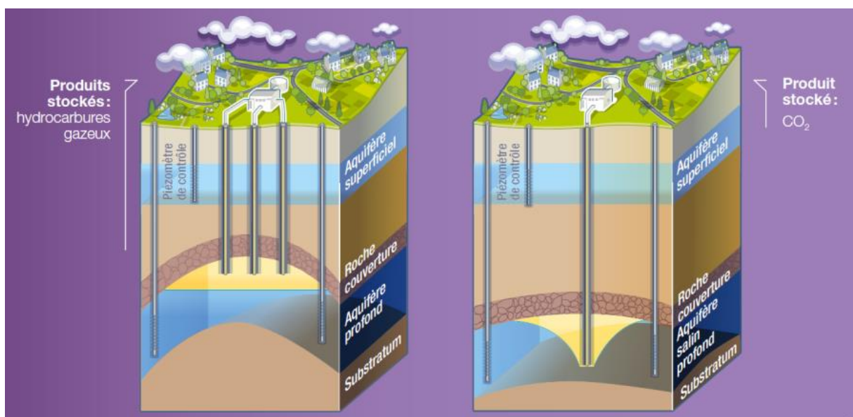
Figure 2. Représentation schématique des stockages en aquifère profond
