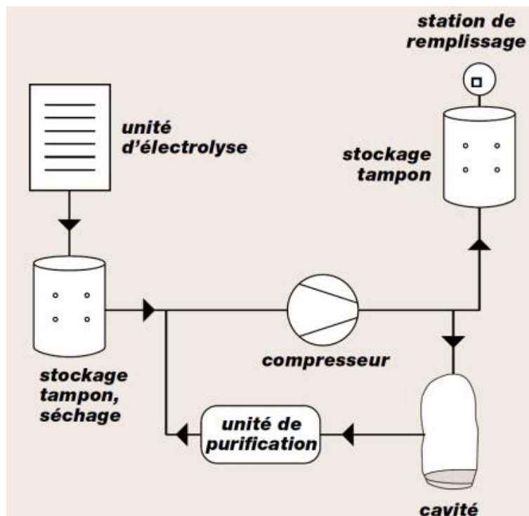
Figure 5. Schéma simplifié des installations d'un stockage souterrain d'hydrogène
