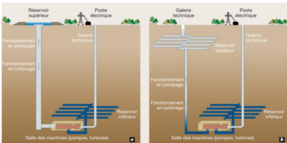
Figure 7. Schéma de principe de l'utilisation d'anciennes mines souterraines comme STEP semi-souterraine (a) et souterraine (b)
