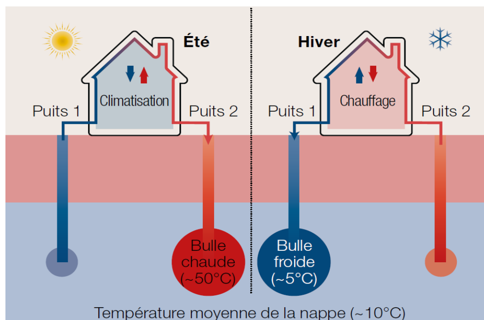
Figure 8. Schéma de principe d'un stockage souterrain d'énergie thermique en aquifère
