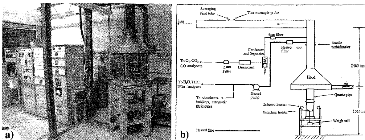
Fig. 2 : Tewarson Calorimeter
