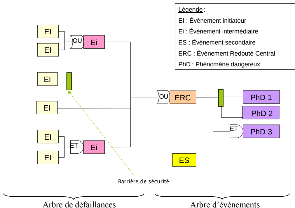
Figure 2 : Nœud papillon
