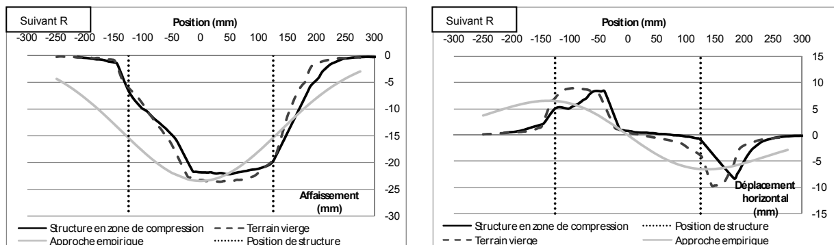
(c) Déplacements vertical et horizontal du terrain - Position 3 (zone de compression)
