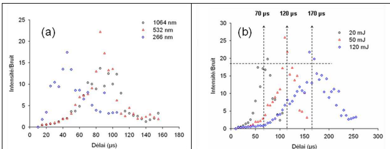
Figure 2. Evolution temporelle du signal LIBS (a) pour trois longueurs d'onde laser différentes, E_{\text{laser}} = 120 \text{ mJ} , \lambda = 1064 \text{ nm} et (b) pour trois énergies laser différentes, argon comme gaz ambiant et \lambda = 1064 \text{ nm} .
