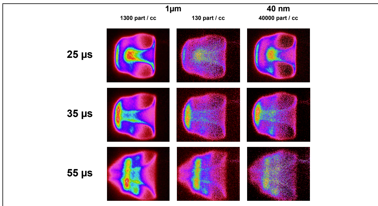
Figure 1. Evolution temporelle de la matière vaporisée (raie du sodium à 588.9 nm) pour deux flux de particules monodispersés de tailles 40 nm et 1 µm.
