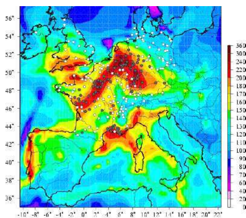
Figure 4 : Simulation du modèle CHIMERE des concentrations d'ozone durant les épisodes de canicules de 2003.
