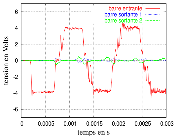
FIG. 2 – Signaux enregistrés
