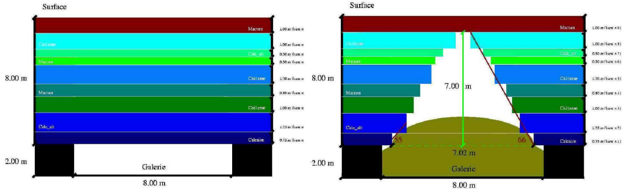
FIG. 4 – Présentation géométrique de la cavité et des matériaux du toit (configuration de la galerie) à gauche. Exemple de remonté de fontis obtenus avec PRF2P.
