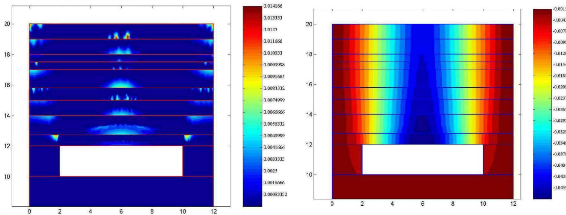
FIG. 5 – Distribution de la plasticité (gauche) et isovaleurs du déplacement vertical (droite). Calculs par éléments finis (EF)
