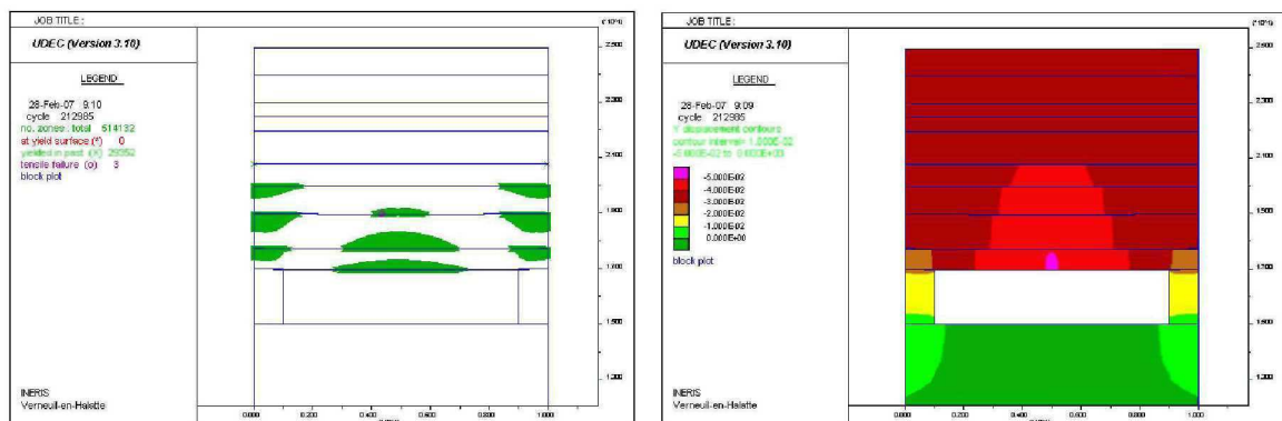
FIG. 6 – Distribution de la plasticité (gauche) et isovaleurs du déplacement vertical (droite). Calculs par différences finis (DF).
