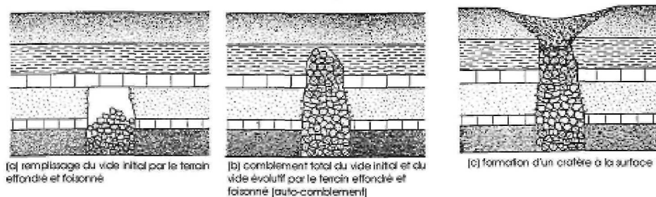
FIG. 2 – Schématisation de la cinétique de formation d'un fontis débouchant au jour
