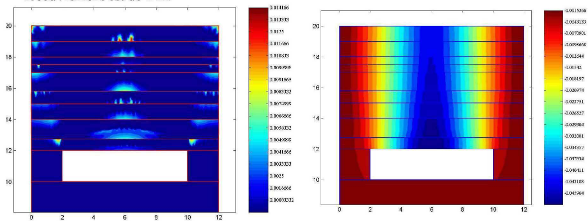
FIG. 5 – Distribution de la plasticité (gauche) et isovaleurs du déplacement vertical (droite). Calculs par éléments finis (EF)
