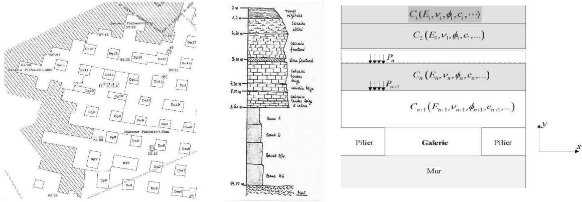
FIG. 3 – Vue en plan d’une carrière souterraine et coupe lithologique du recouvrement (à gauche). Coupe schématique du recouvrement stratifié utilisé dans la construction du modèle numérique PRF2P (à droite).
