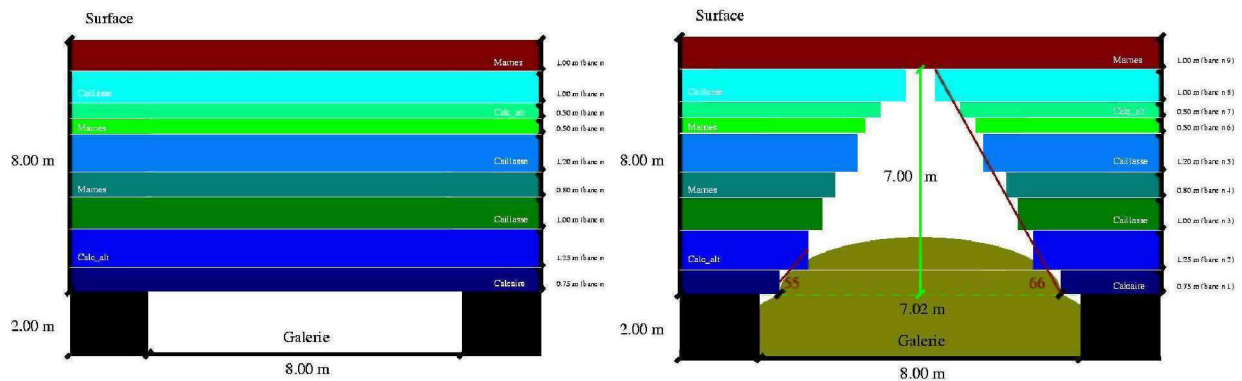
FIG. 4 – Présentation géométrique de la cavité et des matériaux de toit (configuration de la galerie) à gauche. Exemple de remonté de fontis obtenu avec PRF2P.
