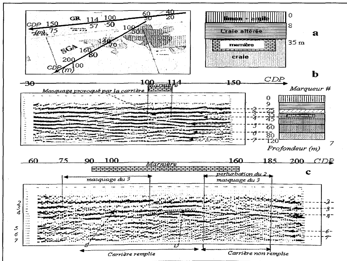
Fig.1.Site St Gilles a) positions des profiles et limites de la carrière; b) Section sismique du profil GR et son interprétation ; c) Section sismique du profil SGA et son interprétation.
