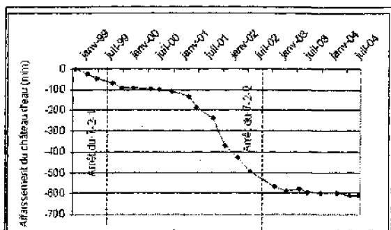
Figure 5 : Profil moyen d'affaissement de douze points de mesures
