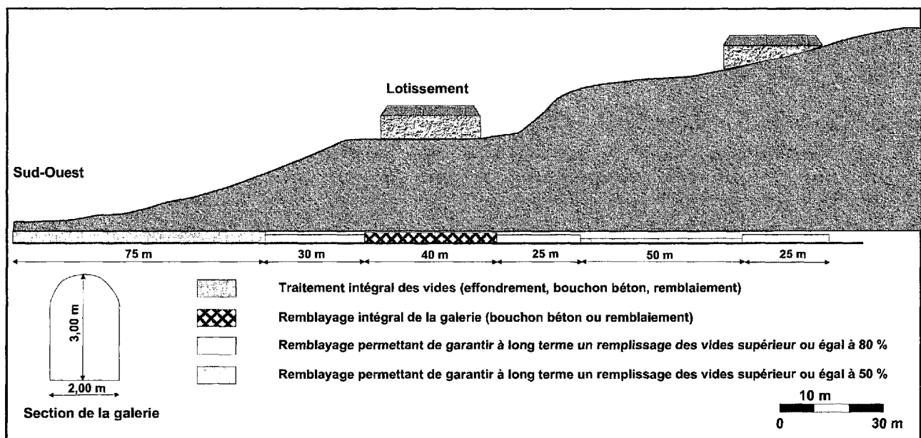
Figure 3 : Principe de traitement de la galerie Saint-Joseph
