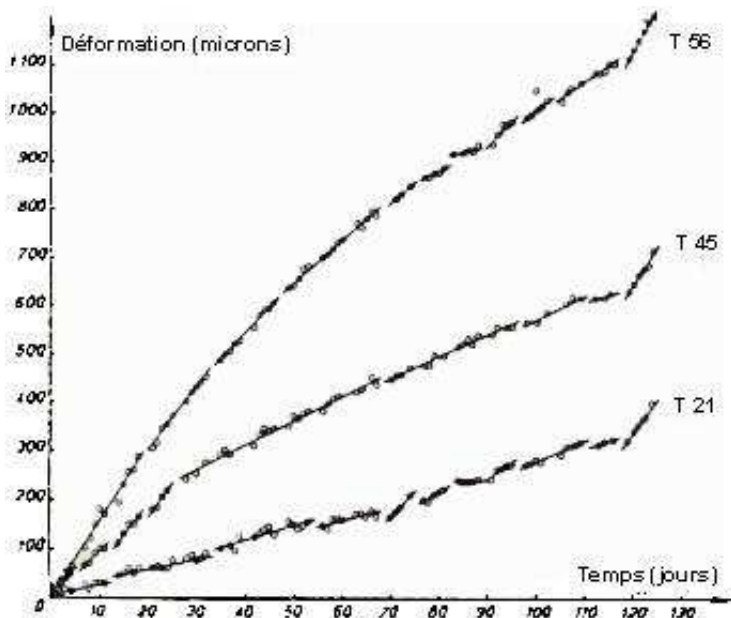
Figure 2 – Surveillance de l’effondrement à partir du fond. Exemple de la mine de fer de Rochonvillers (57), (Josien, 1977) : (a) localisation des cannes de convergence, (b) évolution des mesures de convergence dans le temps.
