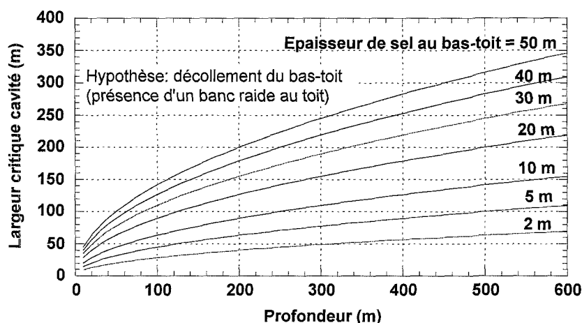
Figure 8 : Estimation de la largeur critique des cavités conduisant à la rupture du toit immédiat détaché d'un banc raide (toit assimilé à une poutre doublement encadrée).
