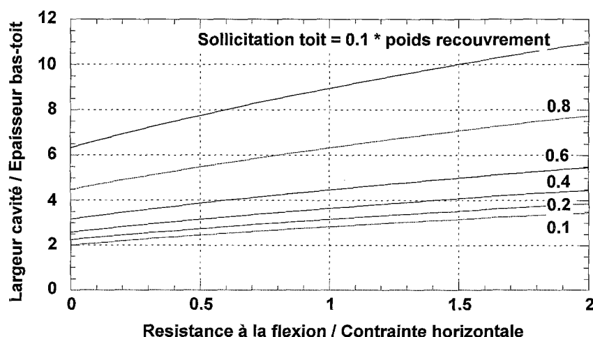
Figure 9- Evaluation de la stabilité du bas-toit soumise à une fraction ou à la totalité du poids du recouvrement (toit assimilé à une poutre doublement encadrée).
