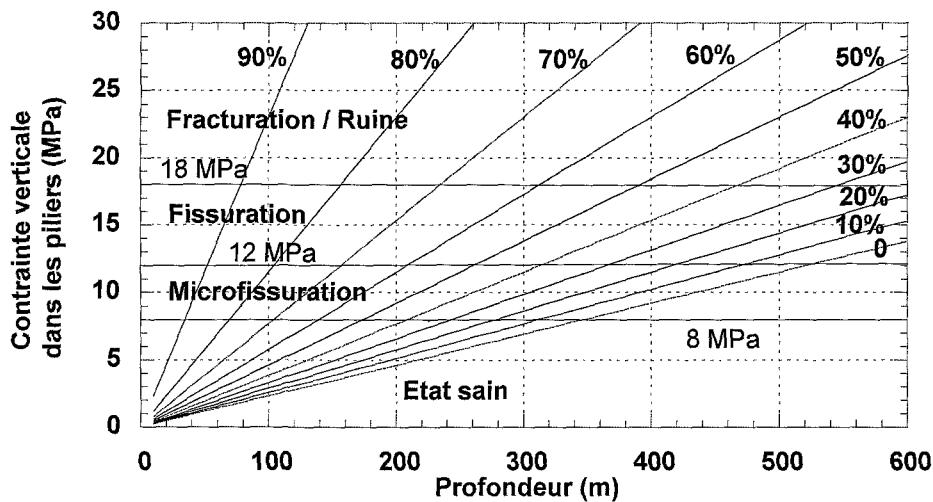
Figure 6 : Evaluation de la stabilité mécanique des piliers dans une exploitation de sel par la méthode de chambres et piliers abandonnés (hypothèse de l'aire tributaire)
