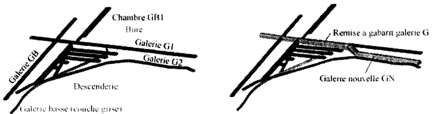
Figure 5 : Modélisation géométrique 3D des ouvrages miniers existants et des nouveaux ouvrages de captage et d'évacuation des eaux de mine.
