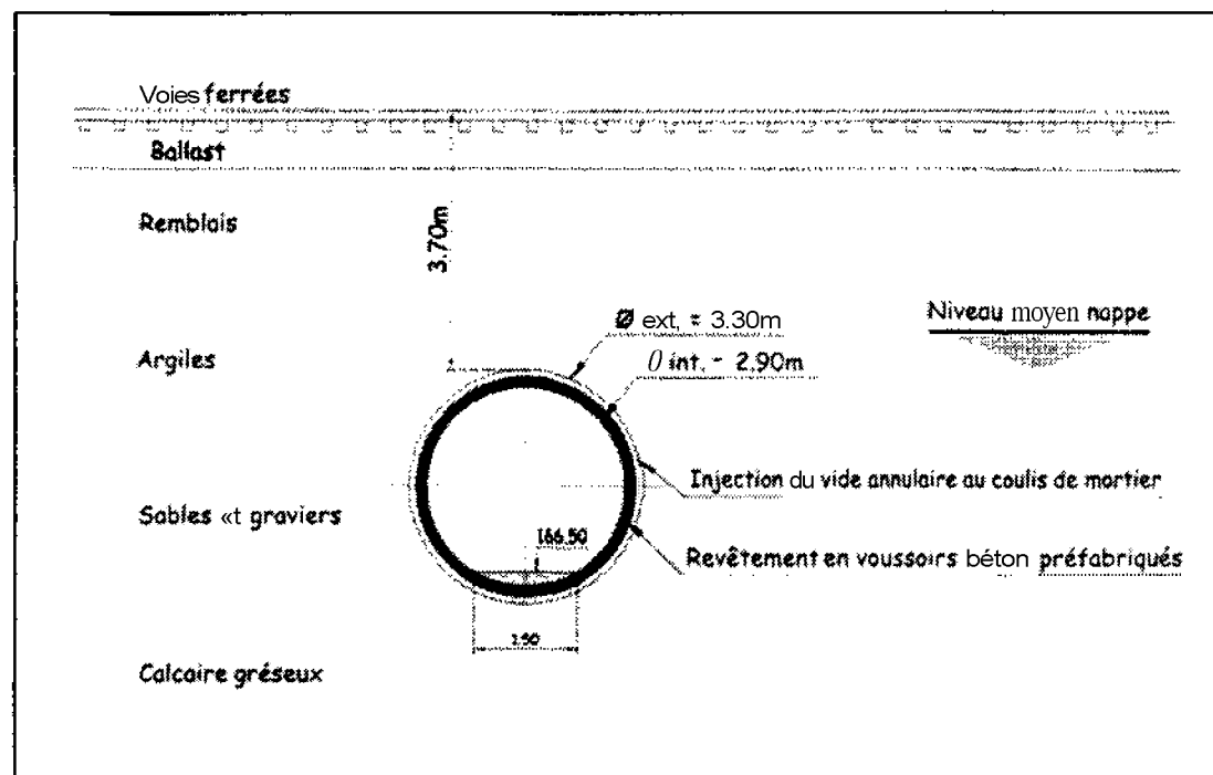
Figure 9 : Coupe de l'ouvrage sous voies ferrées
