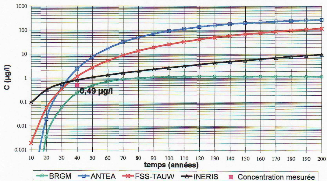
Figure 5 - Simulation de la concentration en naphthalène d'un piézomètre de la craie
