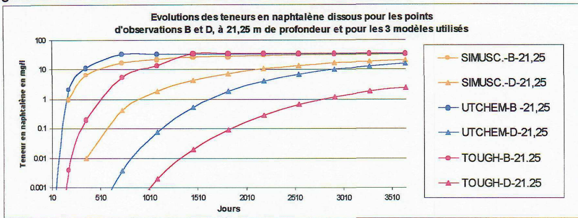
Figure 3 - Courbes de restitution des concentrations en naphthalène dissous simulées dans l'eau en fond de nappe par SIMUSCOPP, UTCHEM et TOUGH2/T2VOC
