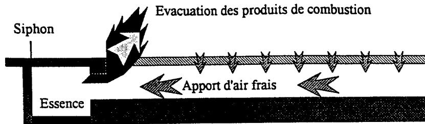
Figure 7 - Schématisation des flux entre le caniveau et le siphon
