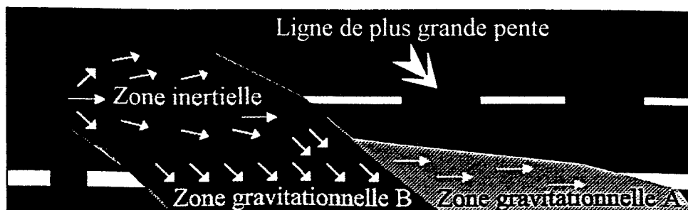
Figure 2 - Schématisation des zones d'écoulement
