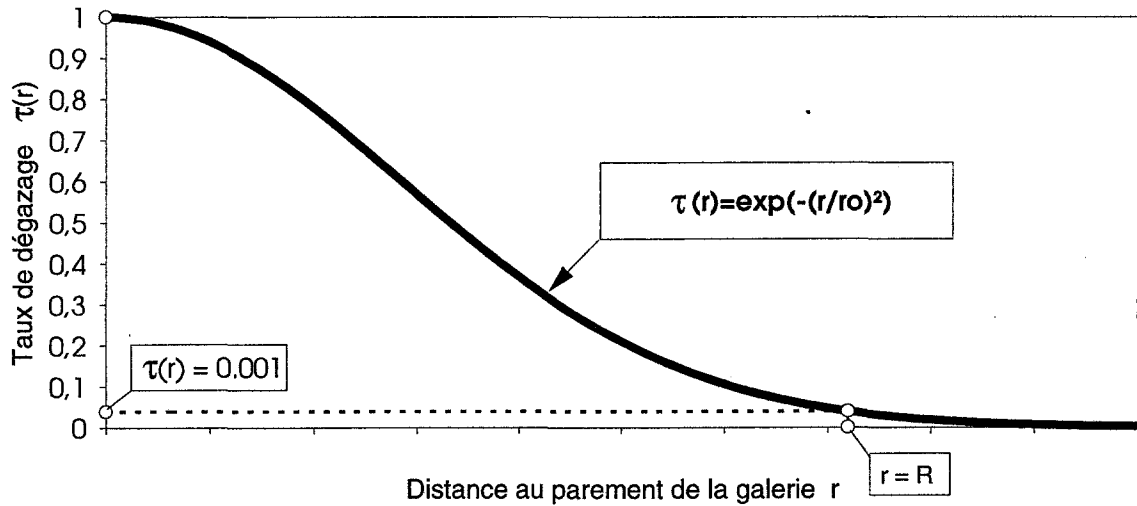
Fig.4. Variation du taux de dégazage en fonction de la distance au parement de la galerie
