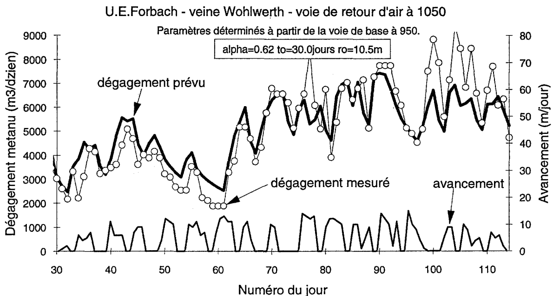
Fig.8. Exemple de prévision avec des paramètres déterminés sur un chantier de référence situé dans la même veine.
