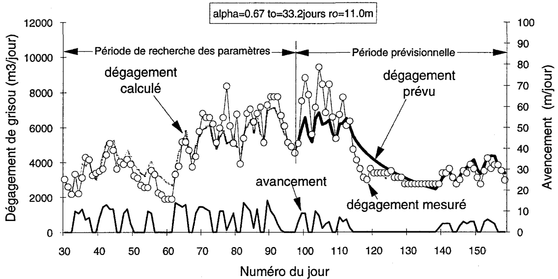
Fig.10. Exemple de prévision pour la suite de traçage avec des paramètres déterminés sur la première partie de la même voie.
