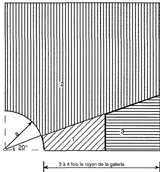
Fig 5 : Limite de la zone où la contrainte axiale \sigma_z est une contrainte majeure pour un rapport de contrainte K = 2
