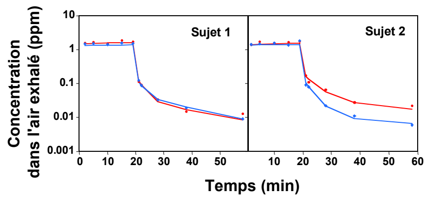
Figure 11 : Prédictions d'un modèle toxicocinétique pour le butadiène calibré à partir de mesures prélevées chez deux sujets en deux occasions différentes. Les mesures et les prédictions associées sont représentées dans une même couleur.
