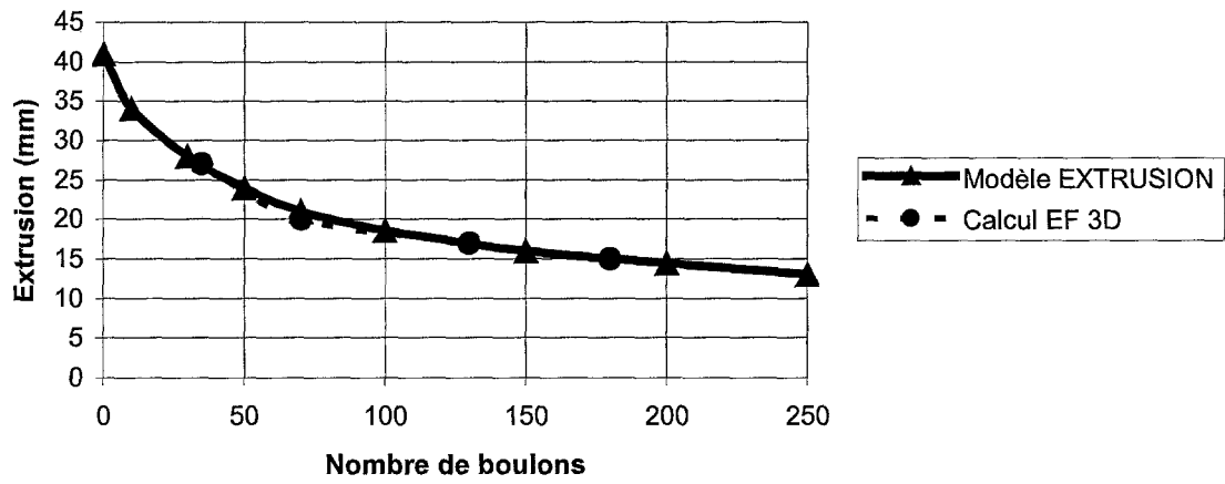
Figure 9 : Comparaison entre le modèle Extrusion et les calculs EF 3D Comparison between the Extrusion model and 3D FEM calculations
