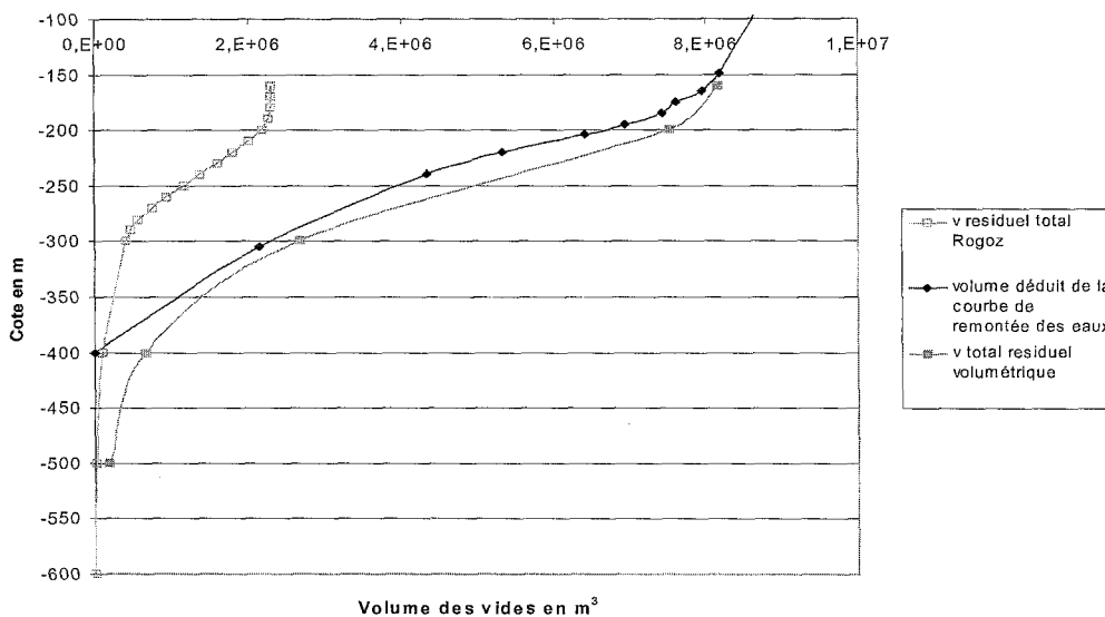
Figure 4. Comparaison entre la répartition selon la profondeur des volumes des vides résiduels cumulés par la méthode empirique de M. Rogoz (1978), par la méthode volumétrique et par le volume mesuré d'après la remontée de l'eau.
