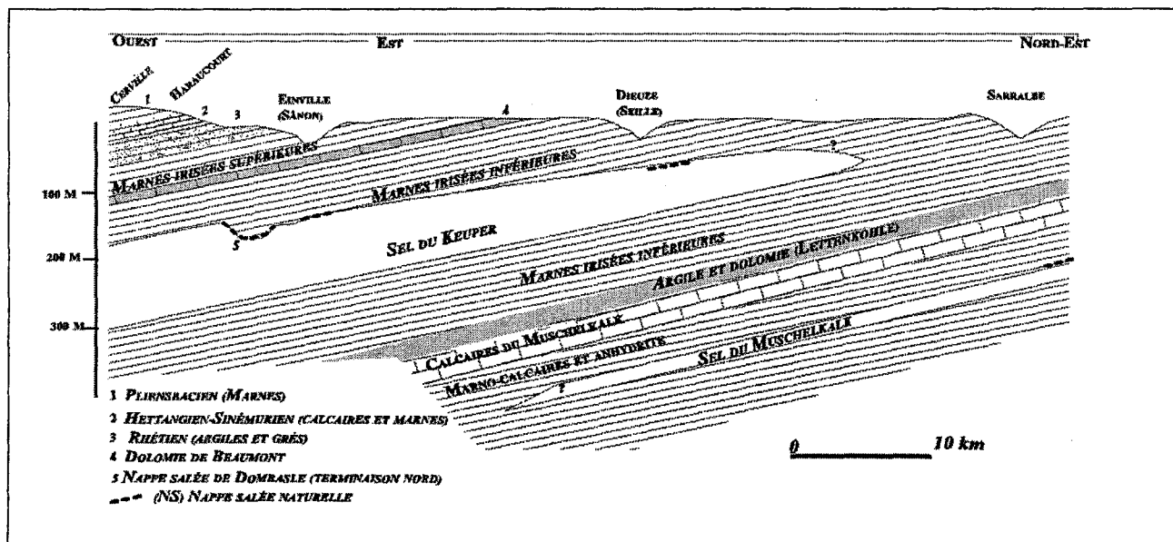
Figure 2 : Coupe géologique schématique des gisements de sel lorrains passant par les principales zones d'exploitation.
