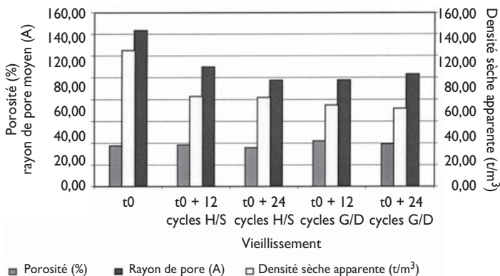
Figure 3 : Évolution moyenne (H, M et B) de la porosité (%), du rayon de pore moyen (Å), et de la densité sèche apparente (t/m 3 ) avant (t0) et après les phases de vieillissement accéléré H/S et G/D (t0 + 12 cycles et t0 + 24 cycles)
