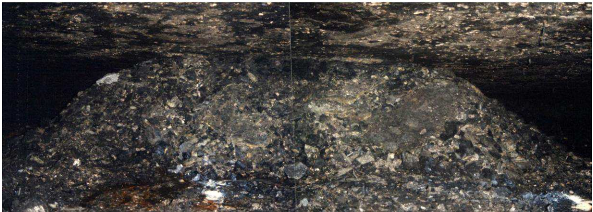
Figure 8 : Pilier de charbon ruiné au sein d'un ancien quartier profond. Figure 8 : Crushed coal pillars within an old mining sector.
