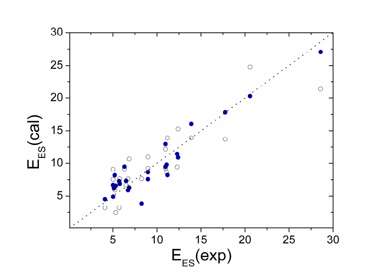
Figure 5 - Sensibilités électriques (en J) calculées selon l'équation (EQ4) (cercles pleins bleus) et selon le modèle de Keshavarz [26] (cercles vides) en fonction des valeurs expérimentales
