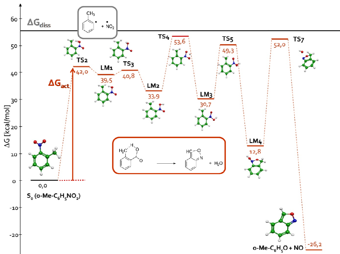
Figure 6 - Mécanismes de décomposition de l'ortho-nitrotoluène calculés à l'aide de la DFT [28]
