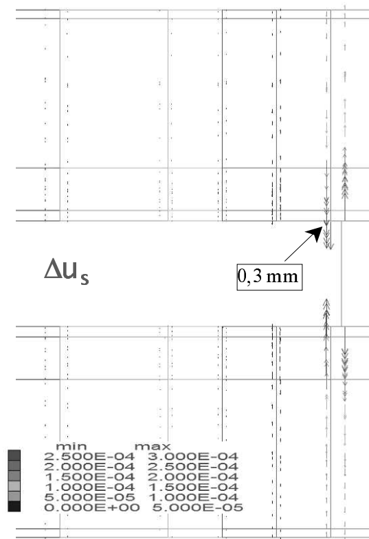
b - Déplacements tangentiels des failles
