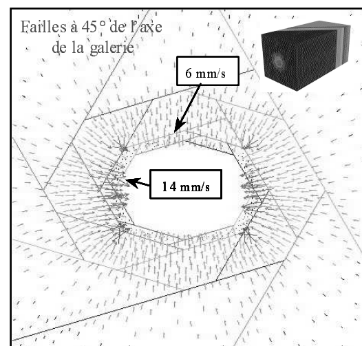
Figure 8 : Impact de l'orientation des fractures sur les profils verticaux d'ouverture hydraulique dans les fractures les plus proches du front de creusement de la galerie et sur la distribution des vitesses d'écoulement dans la fracture la plus éloignée du front (traits pointillés : fracture à 90^\circ axe galerie ; traits pleins : fracture à 45^\circ axe galerie)
