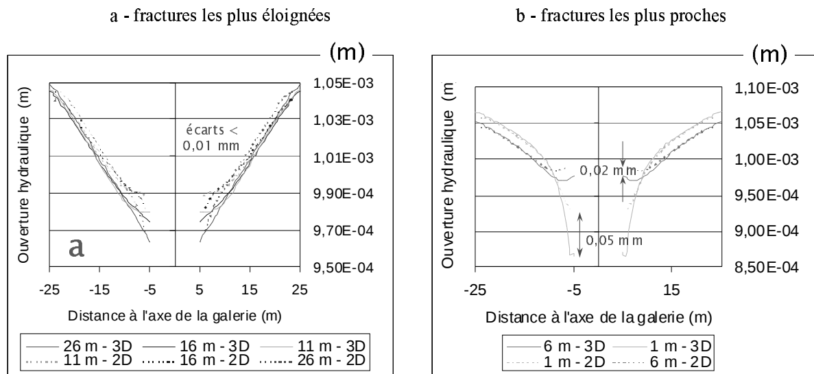
Figure 3 : Comparaison des profils verticaux d'ouverture hydraulique obtenus avec UDEC (traits pointillés) et 3DEC (traits pleins) dans les 5 fractures.
