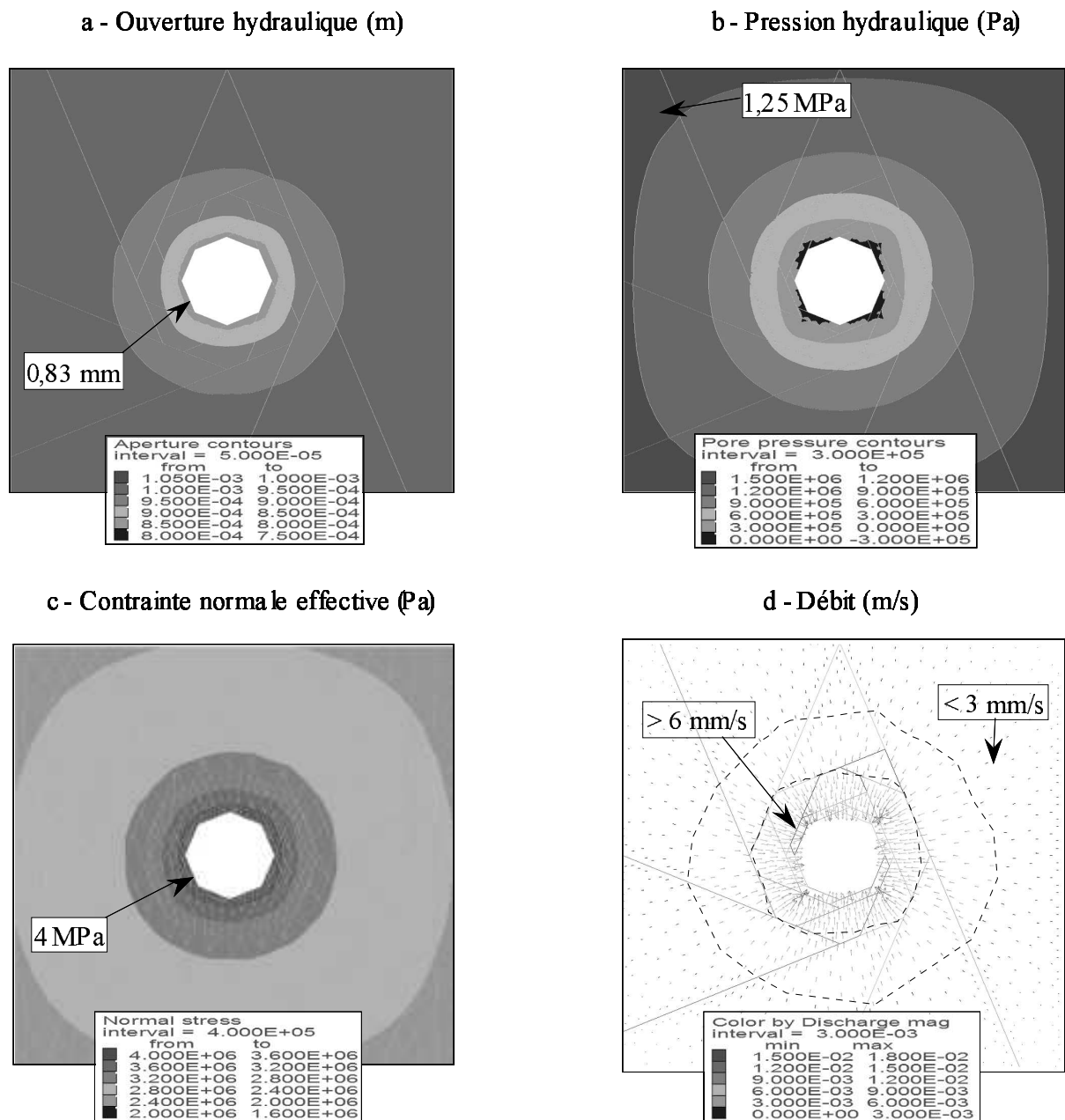
Figure 6 : Isovaleurs d'ouverture hydraulique (a), de pression hydraulique (b), de contrainte normale effective (c) et distribution des vitesses d'écoulement dans la fracture la plus proche du front de creusement de la galerie (modèle de référence)
