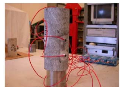
Figure 4. Essais acoustiques en laboratoire, Système d'acquisition
