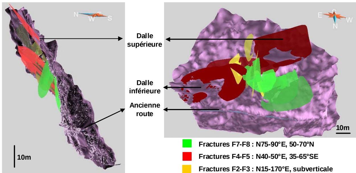
Figure 7. Prolongement du réseau de fractures en profondeur. A gauche : vue de côté, en direction du NE. A droite : vue de derrière
